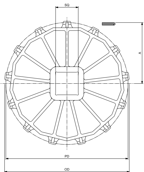
方孔 - 主/被动轮
