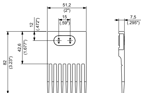
型号 TC611-04
