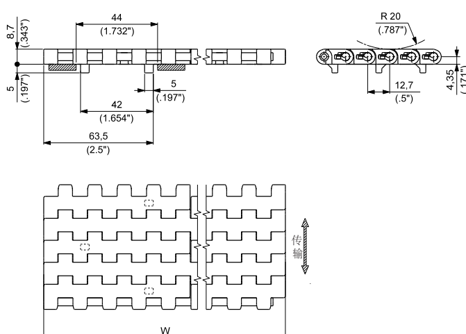
含导块
