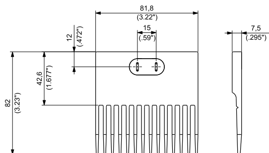
型号 TC611-07
