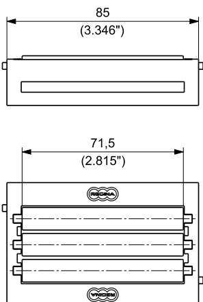
型号 CC000481 (专为 4650 网带系列研发)
