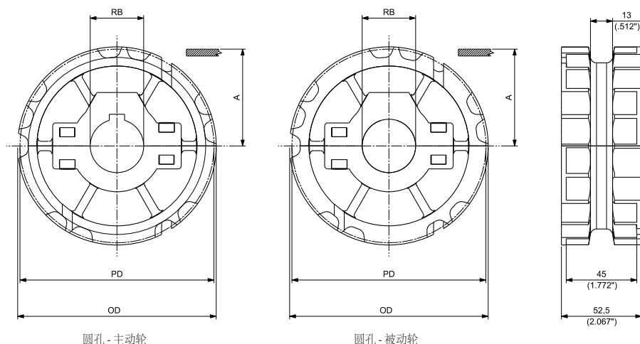
圆孔 - 主动轮
