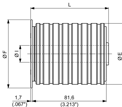
单挡边加长包胶托辊
