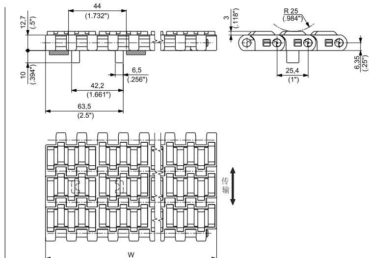
含导块
