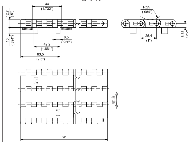
含导块
