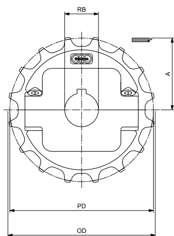
圆孔 - 主动轮
