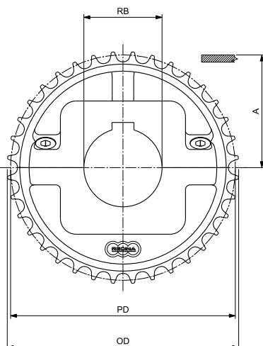
圆孔 - 主动轮
