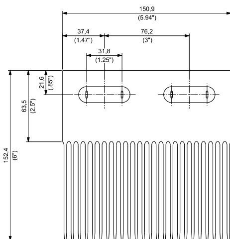
型号 TC3000-01
