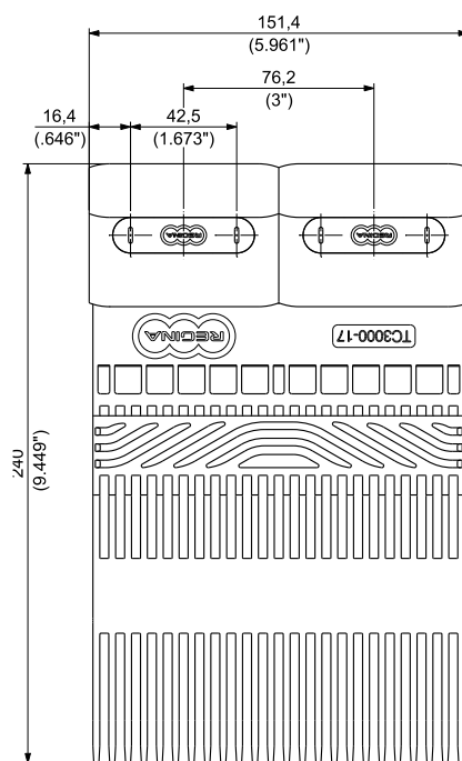
型号 TC3000-17
