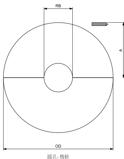
圆孔-惰轮
