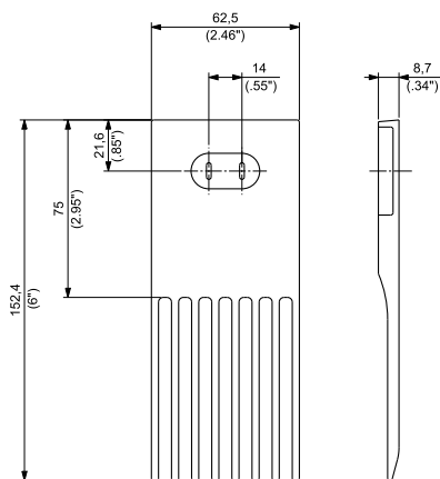
型号 TC1600-01
