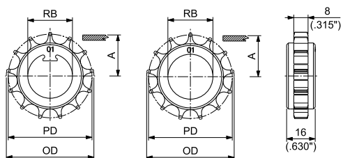
圆孔 - 主动轮
