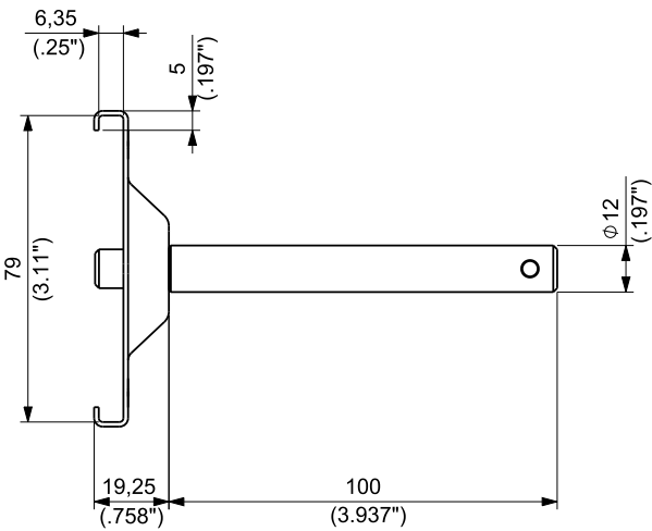
不锈钢夹爪
