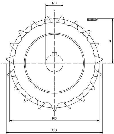
圆孔 - 主动轮
