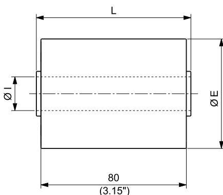
加长托辊
