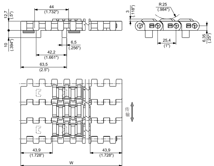
含导块
