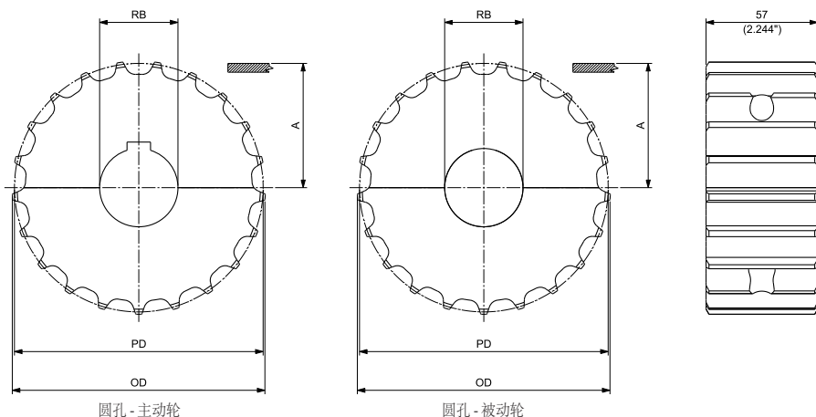
圆孔 - 主动轮
