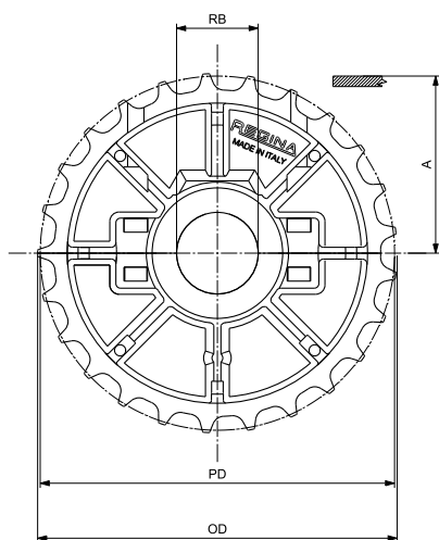
圆孔 - 被动轮
