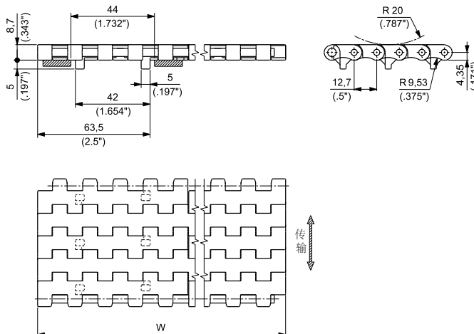
含导块
