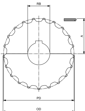
圆孔 - 主动轮
