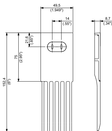
型号 TC1600-03
