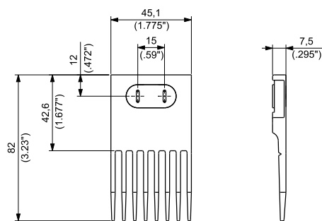
型号 TC611-03
