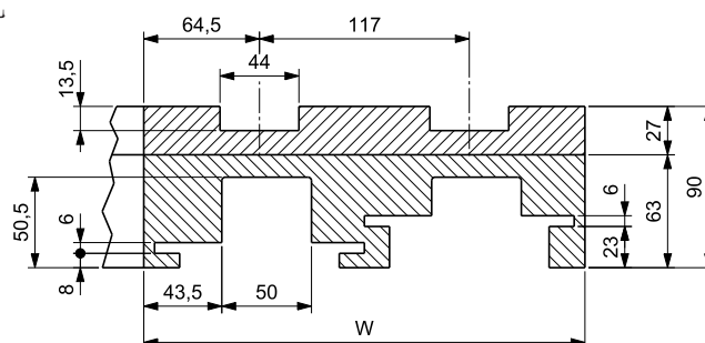
回程导块
