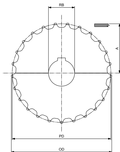
圆孔 - 主动轮
