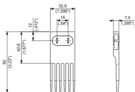
型号 TC611-01
