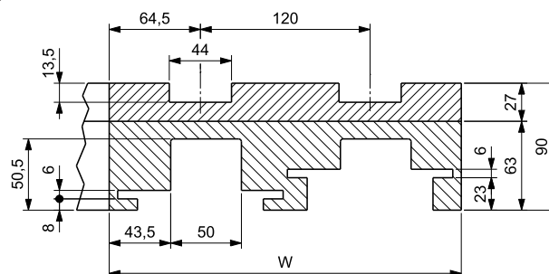
回程导块
