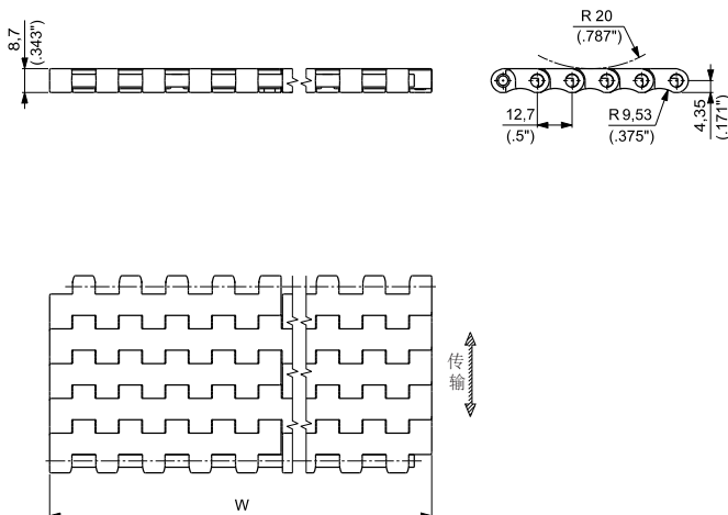
无导块
