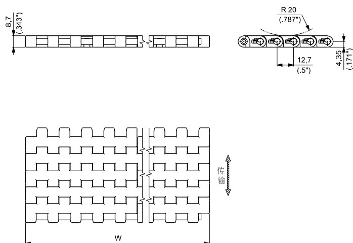
无导块
