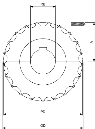
圆孔 - 主动轮
