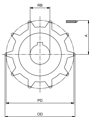
圆孔 - 主动轮
