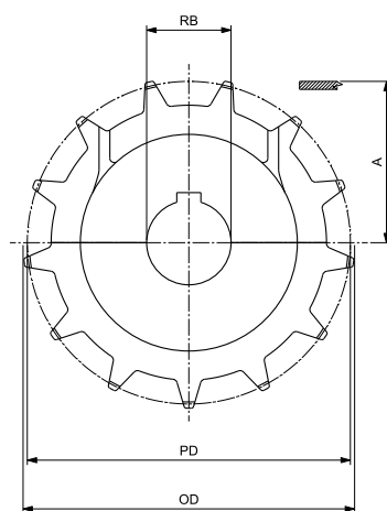
圆孔 - 主动轮
