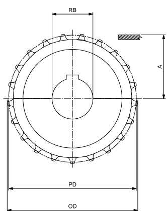
圆孔 - 主动轮
