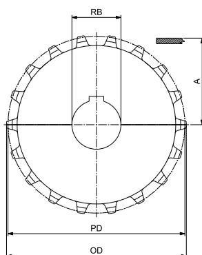
圆孔 - 主动轮
