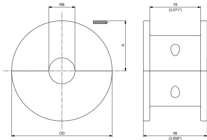
圆孔-惰轮
