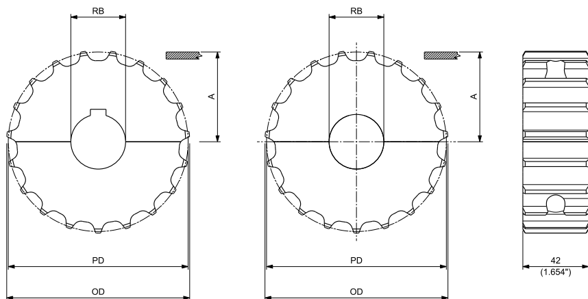
圆孔 - 主动轮
