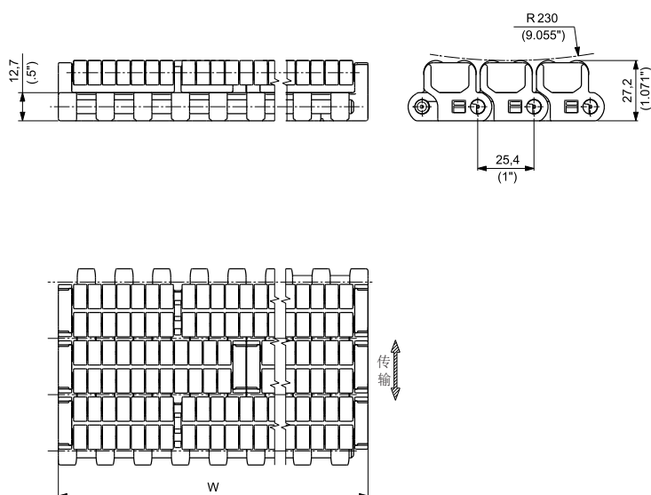
无导块
