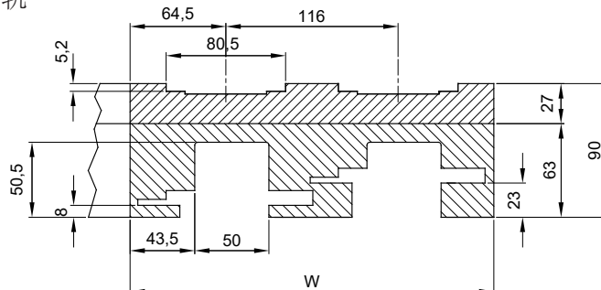
多轨
