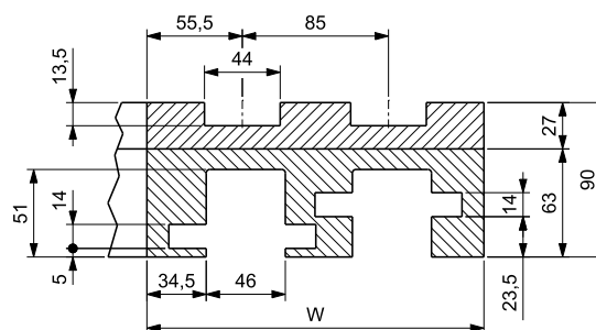
回程导块
