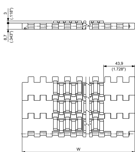
无导块
