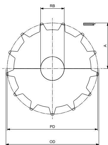
圆孔 - 被动轮
