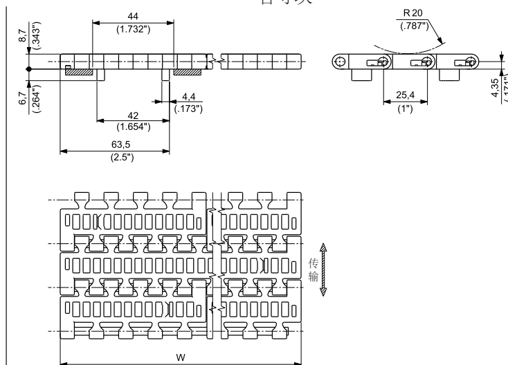
含导块
