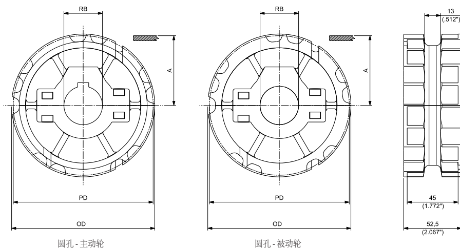
圆孔 - 主动轮
