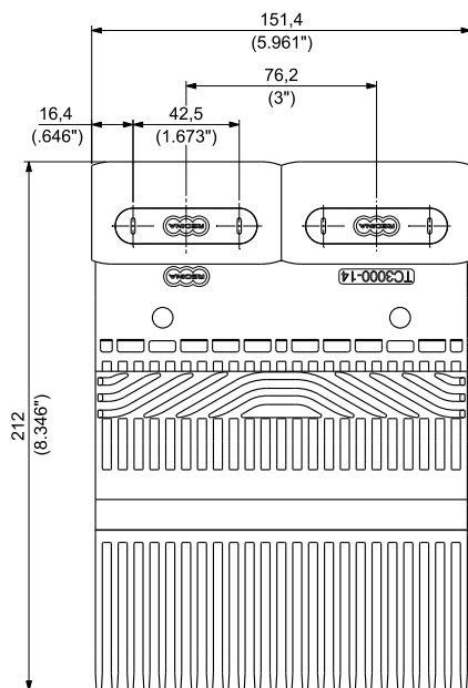
型号 TC3000-14
