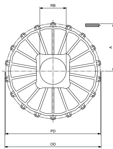
圆孔 - 被动轮
