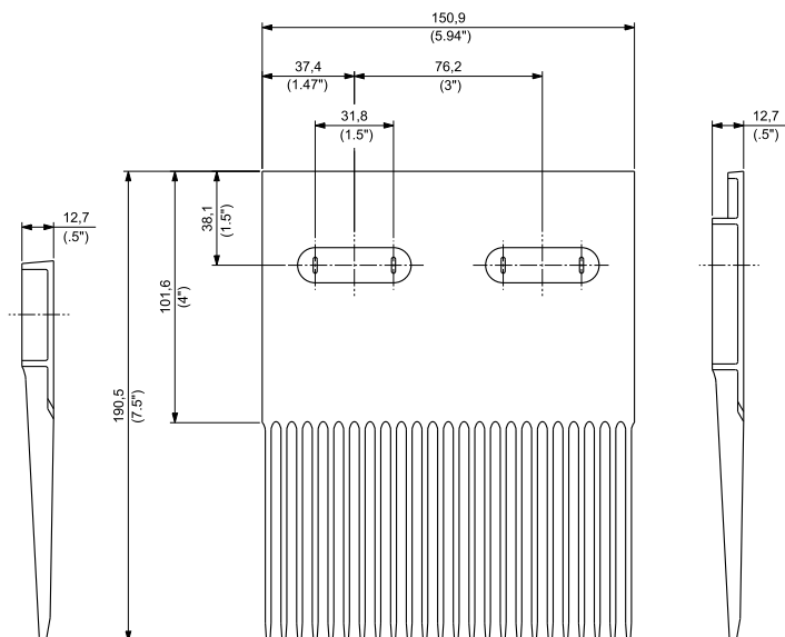
型号 TC3000-02
