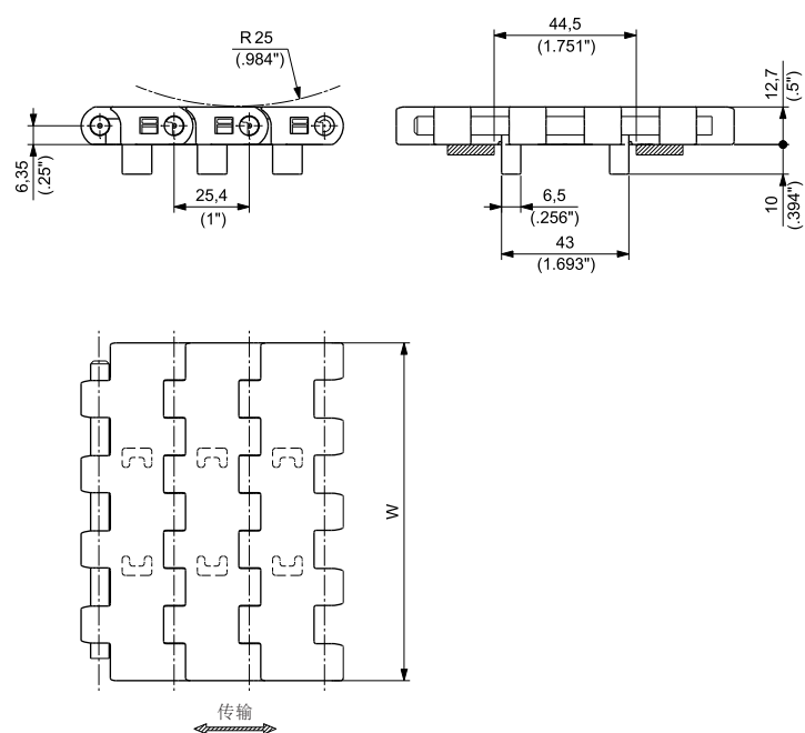
含导块
