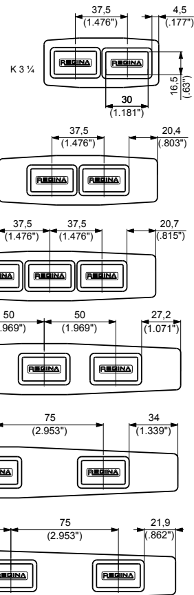
橡胶垫分布
