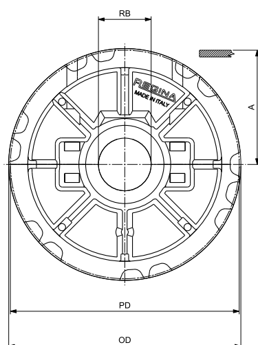
圆孔 - 被动轮
