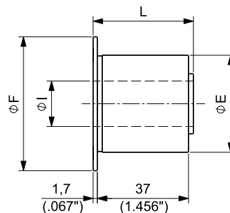
单挡边托辊
