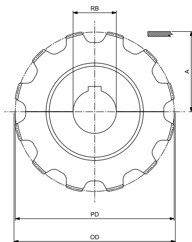
圆孔 - 主动轮
