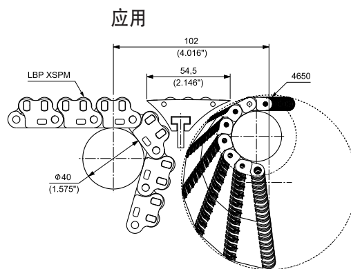
示例安装用于 4650 与 LBP XSPM 网带。 4650 网带与其它网带系列的安装， 请联系雷吉那技术部门。
