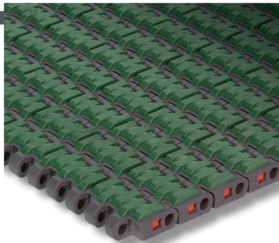
含导块
