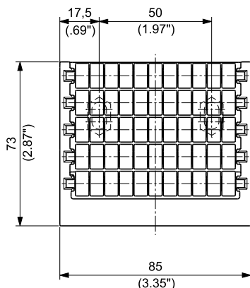
型号 LTP-5RKQ
