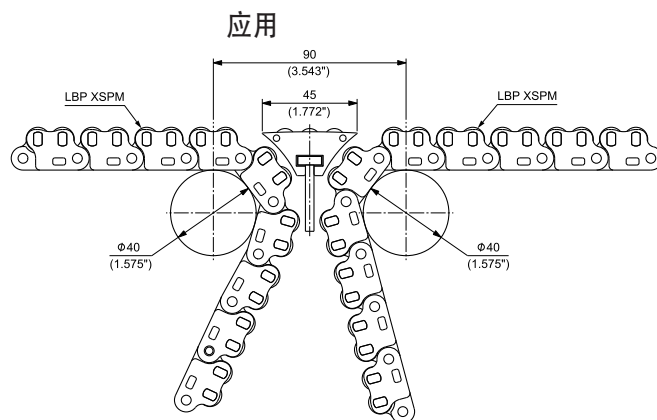
示例安装用于 LBP XSPM 网带。 其它网带系列的安装， 请联系雷吉那技术部门。
