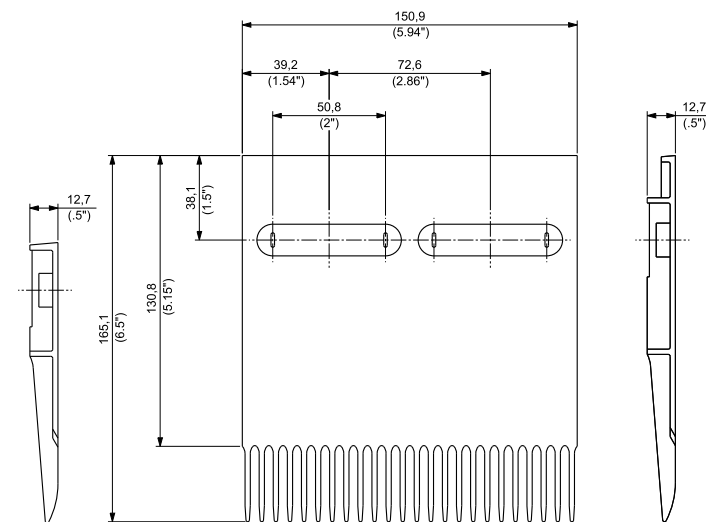
型号 TC3000-04
