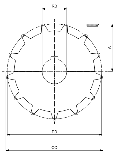
圆孔 - 主动轮
