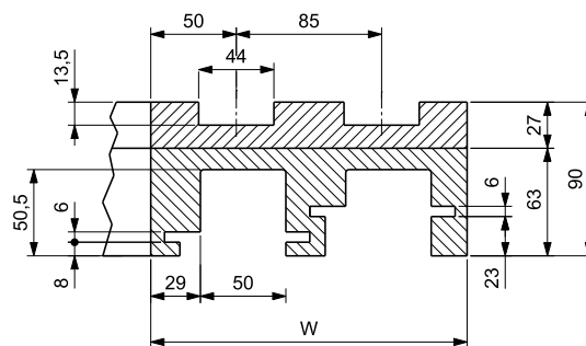
回程导块
