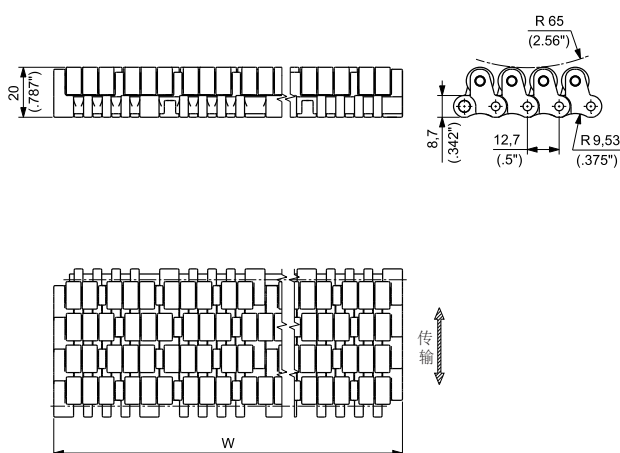
无导块
