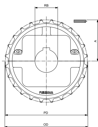
圆孔 - 主动轮
