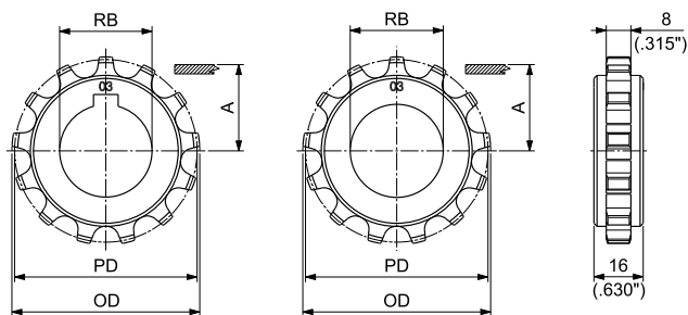
圆孔 - 主动轮
