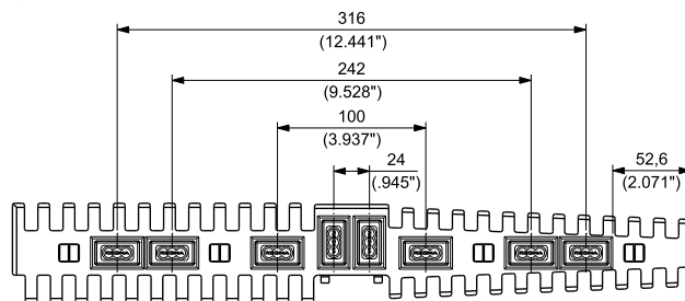
8-胶型
