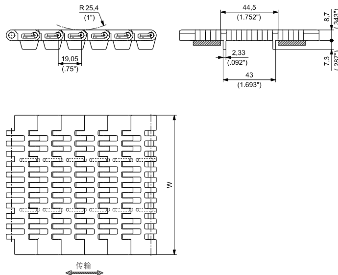
含导块
