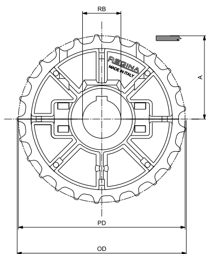
圆孔 - 主动轮
