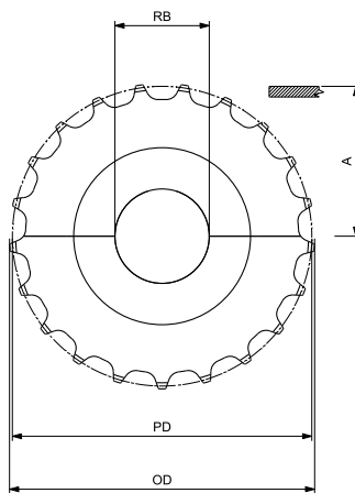
圆孔 - 被动轮
