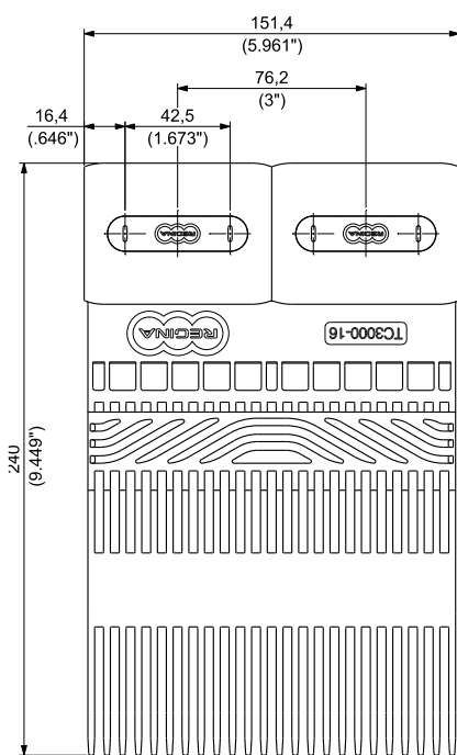
型号 TC3000-16
