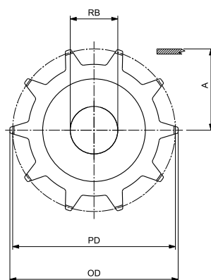
圆孔 - 被动轮
