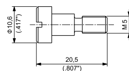
Artikelnummer 16300005
