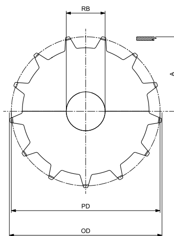
RUNDE BOHRUNG - UMLenkUNG
