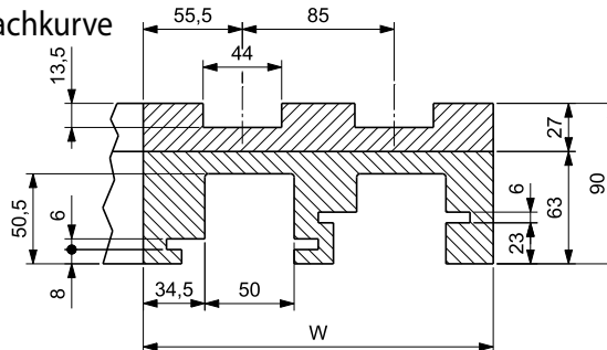
Einlaufschuh
