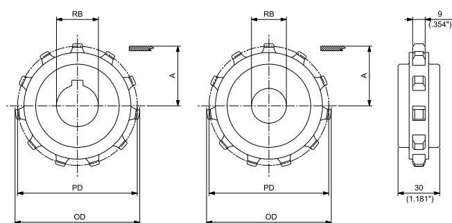
RUNDE BOHRUNG - ANTRIEB
