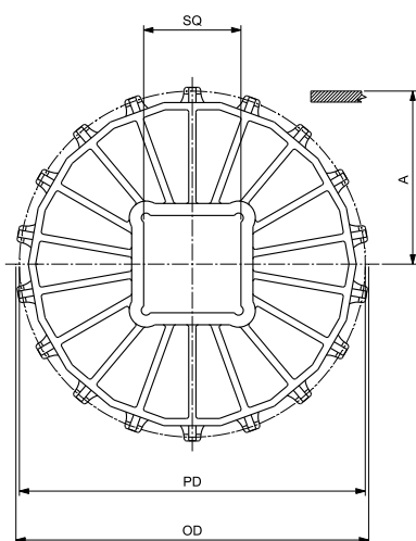
VIERKANTBOHRUNG - ANTRIEB/UMLenkUNG
