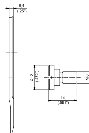
Artikelnummer 16300020
