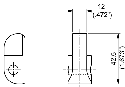
ARTIKELNUMMER: 233/1700
