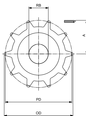
RUNDE BOHRUNG - UMLenkUNG
