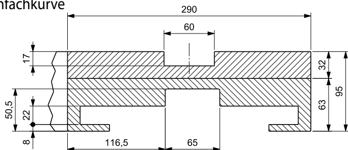
Einfachkurve
