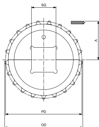
VIERKANTBOHRUNG - ANTRIEB/UMLenkUNG
