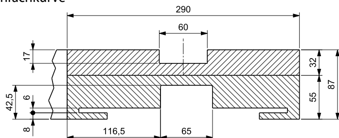
Einfachkurve
