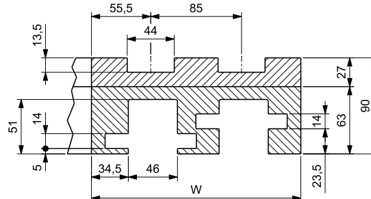
Mehrfachkurve
