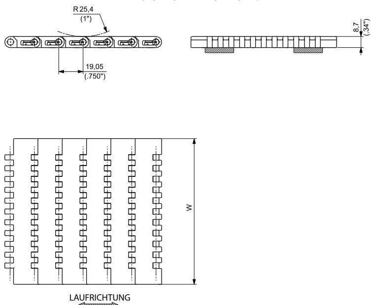
VERSION OHNE FÜHRUNG
