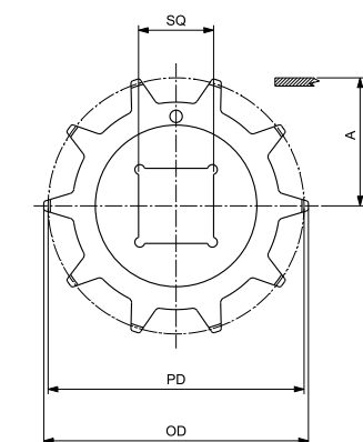
VIERKANTBOHRUNG - ANTRIEB/UMLenkUNG
