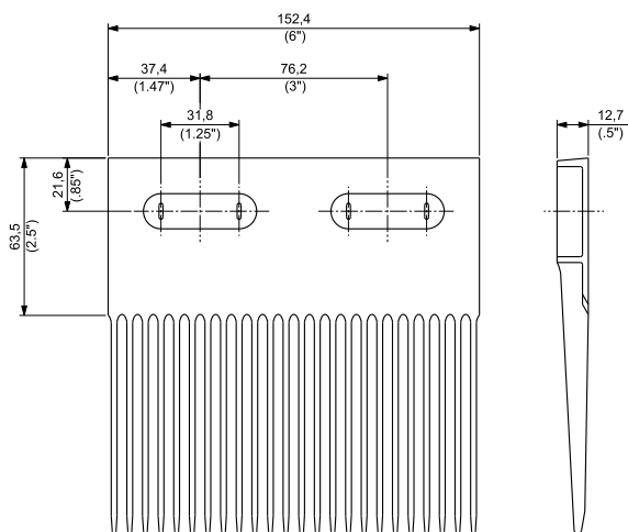
Artikelnummer TC3000-01
