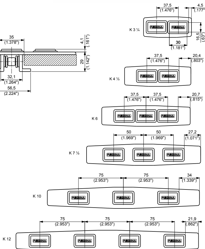
GUMMIPLATTEN-ANORDNUNG
