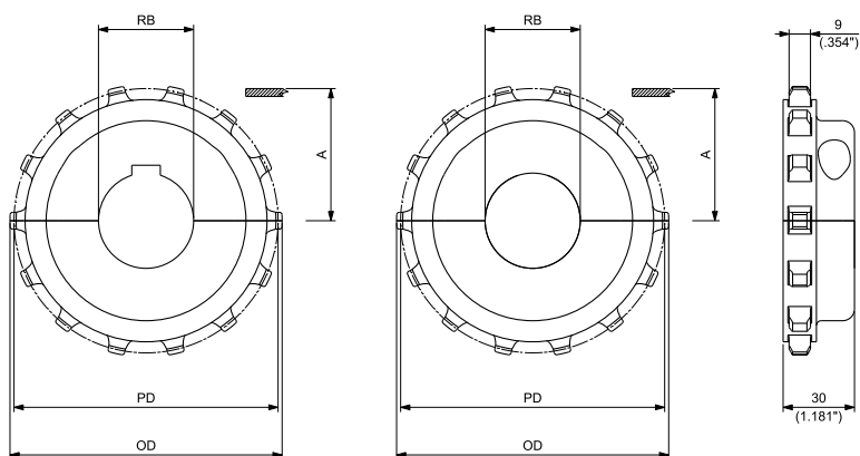
RUNDE BOHRUNG - ANTRIEB
