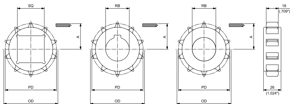
VIERKANTBOHRUNG - ANTRIEB/UMLENKUNG
