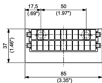
Artikelnummer LTP-2RKQ
