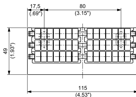
Artikelnummer LTP-3RKG
