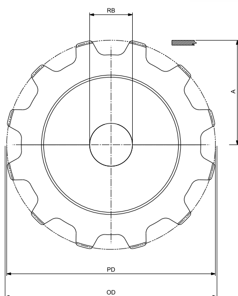
RUNDE BOHRUNG - UMLENKUNG
