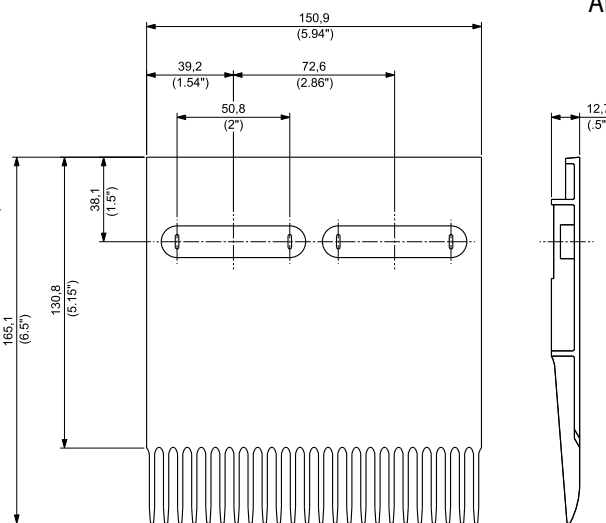
Artikelnummer TC3000-04
