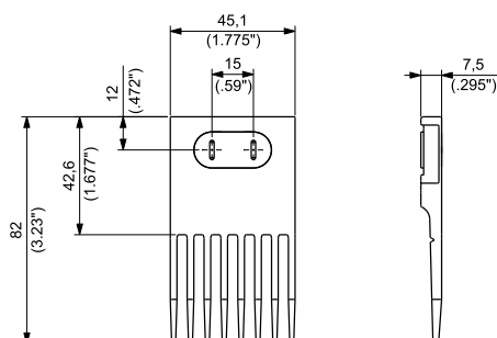
KAMM FÜR K 37 KETTE
