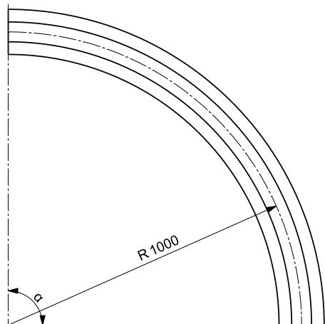
Einlaufschuh
