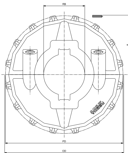
RUNDE BOHRUNG - ANTRIEB
