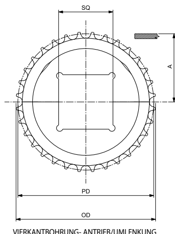
VIERKANTBOHRUNG - ANTRIEB/UMLenkUNG
