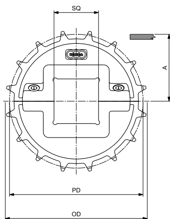
VIERKANTBOHRUNG - ANTRIEB/UMLenkUNG
