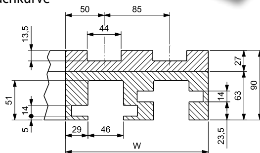
Mehrfachkurve
