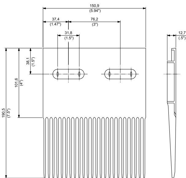
Artikelnummer TC3000-02
