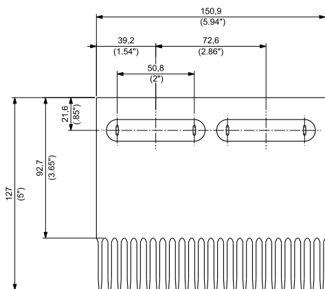
Artikelnummer TC3000-03
