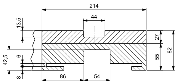
Einfachkurve
