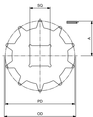
VIERKANTBOHRUNG - ANTRIEB/UMLenkUNG
