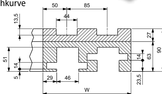
Mehrfachkurve
