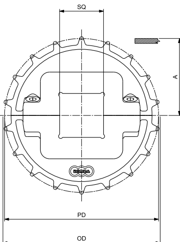
VIERKANTBOHRUNG - ANTRIEB/UMLenkUNG
