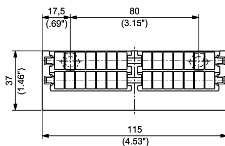
Artikelnummer LTP-2RKG
