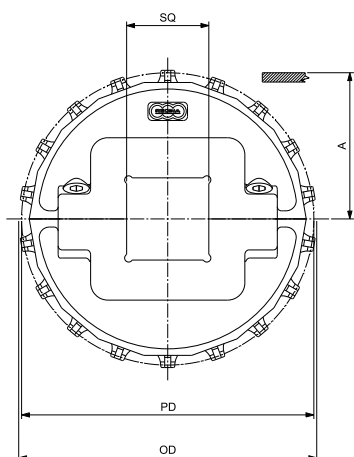
VIERKANTBOHRUNG - ANTRIEB/UMLenkUNG
