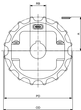
VIERKANTBOHRUNG - ANTRIEB/UMLenkUNG
