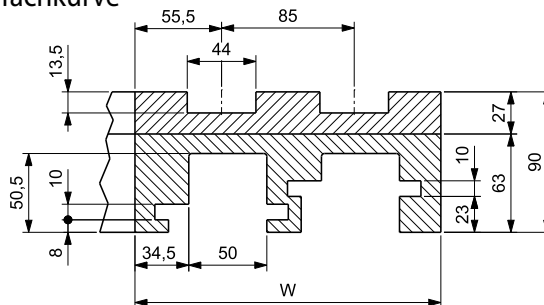
Mehrfachkurve
