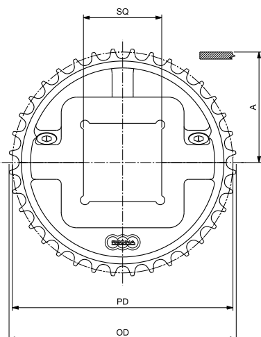
VIERKANTBOHRUNG - ANTRIEB/UMLenkUNG
